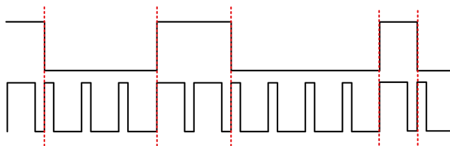
GP9301BM与GP9301B输出信号关系
