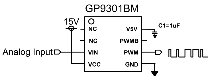
GP9301B 电压转PWM关系
