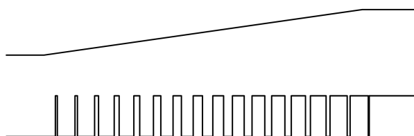
GP9301BM与GP9301B输出信号关系
